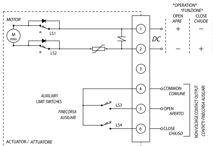
- EXAMPLE OF EXTERNAL CIRCUIT - - ESEMPIO DI CIRCUITO ESTERNO -
